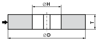
Ściernica do obłuskiwaczy ziarna EKONOS 101 - D \times T \times H
